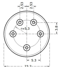
底部尺寸图
