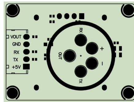
OLED 显示板连接
