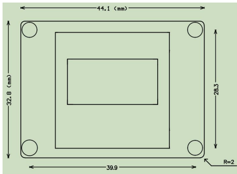
OLED 显示板尺寸
